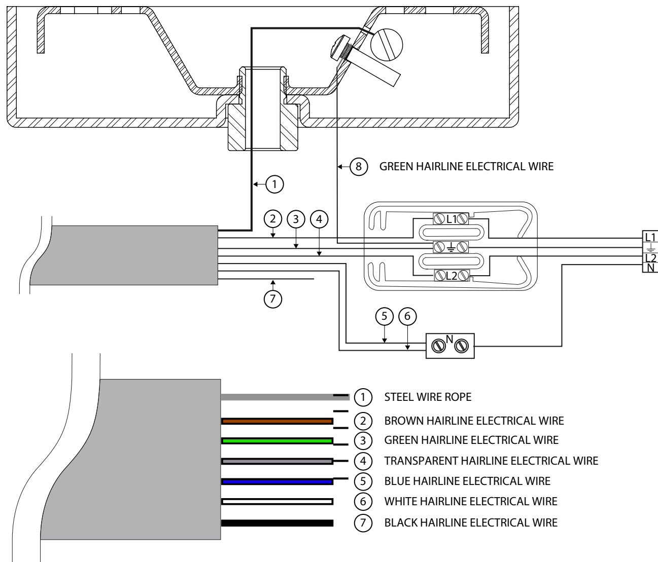
schema elettrico - wiring diagram - schaltplan - schéma de câblage - diagrama de cableado
